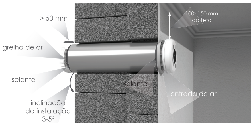
Fig.4 Esquema de instalação do recuperador na parede.
