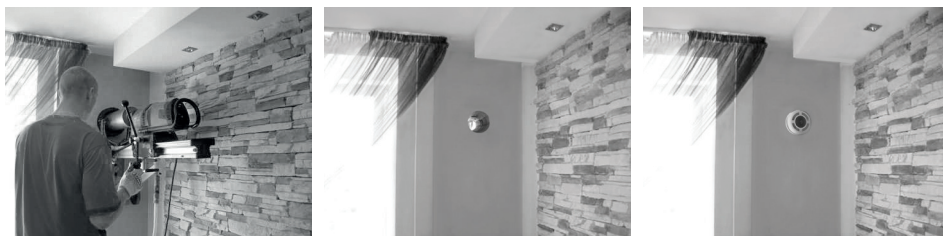
Fig.5 O exemplo de montagem do recuperador PRANA-150, PRANA-200C, PRANA-200G.
