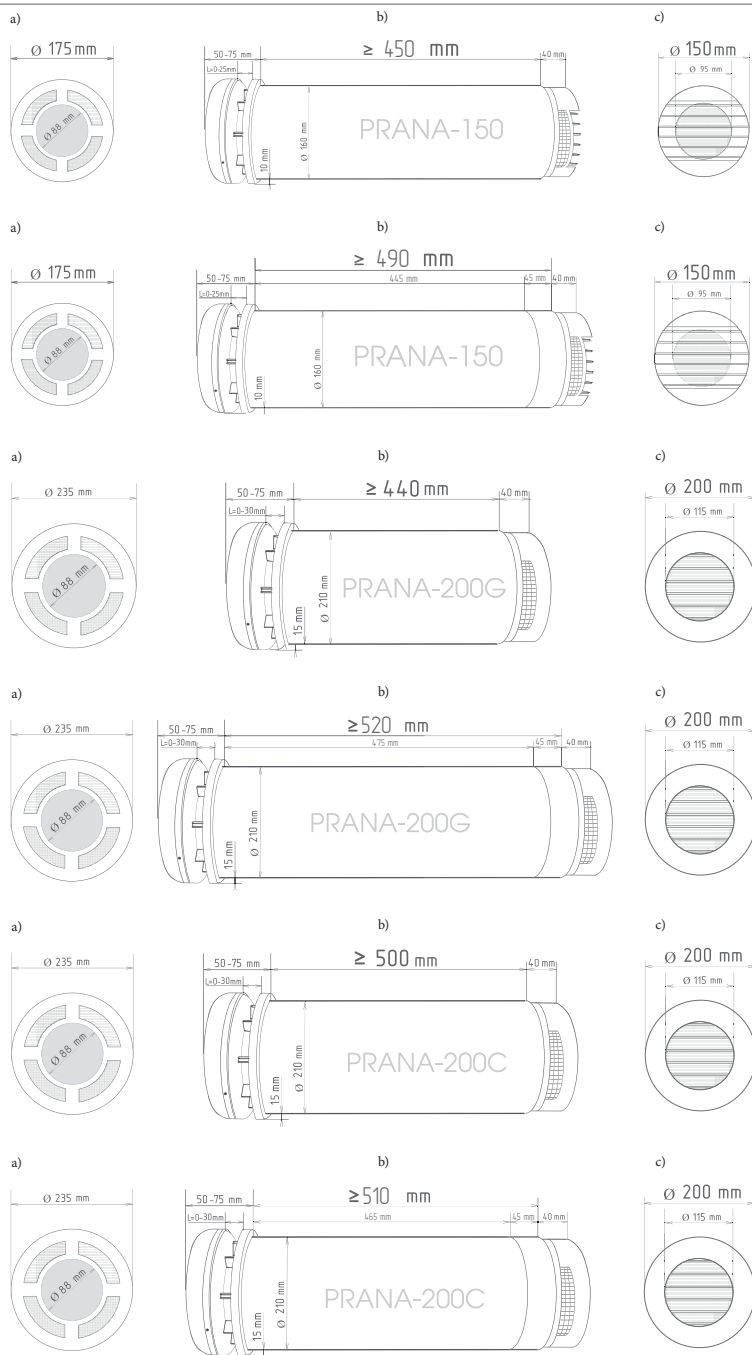
Fig.3 Dimensões e tamanho do sistema de ventilação «PRANA-150», «PRANA-200G», «PRANA-200C»:
